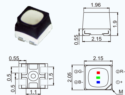
NH-Z1921RGBA-SG 2.15×2.05×1.9
