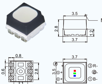
FM-Z3535RGBA-SH 3.7×3.5×2.8
