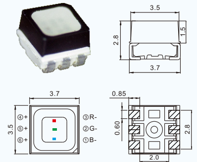
NH-Z3535RGBW-SG 3.7×3.5×2.8
