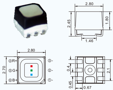
NH-Z2727RGBA-SG 2.8×2.7×2.45
