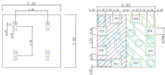
Tolerance: ±0.05mm unit:mm
